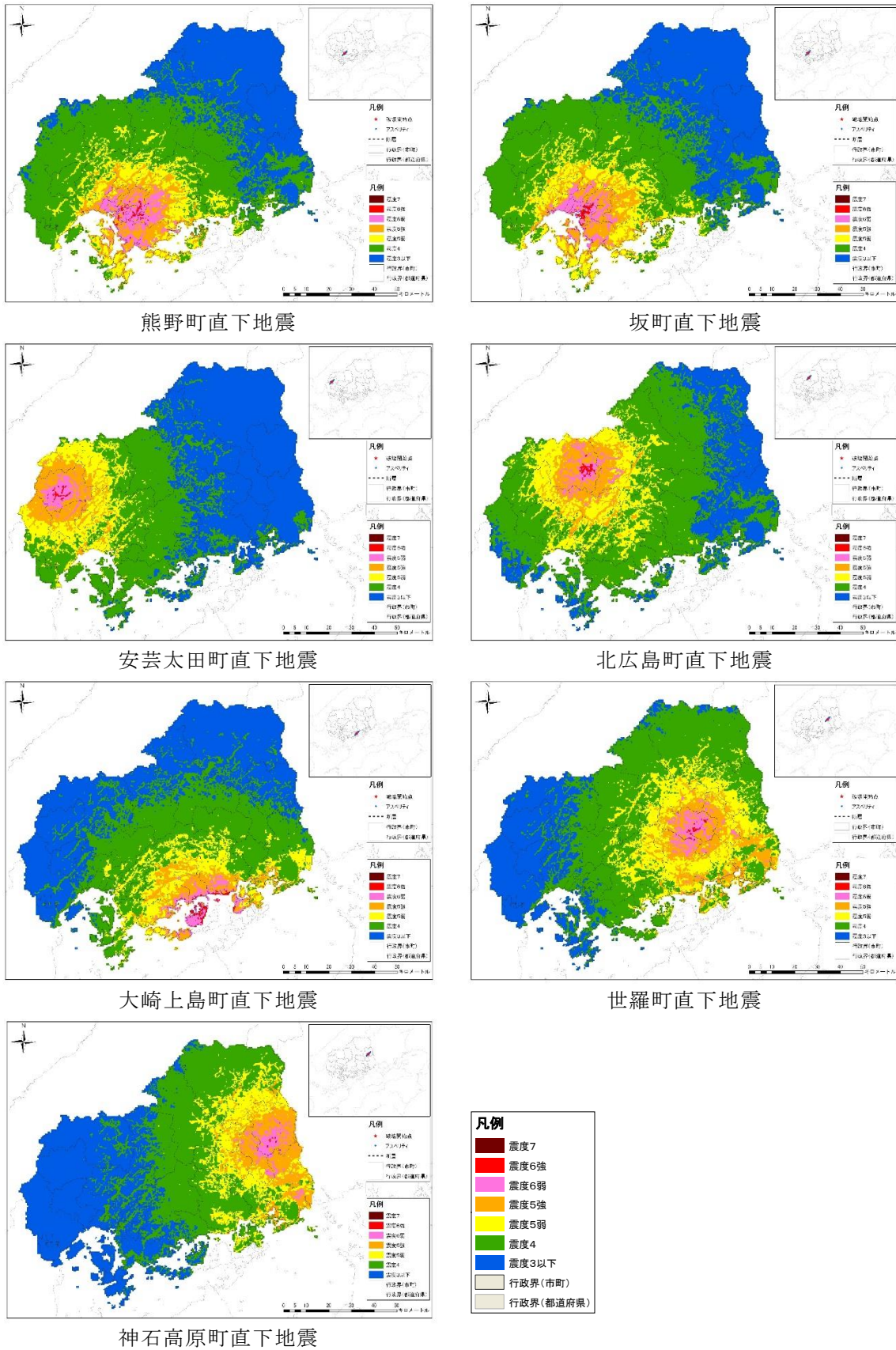
図-4 (5) 震度分布
